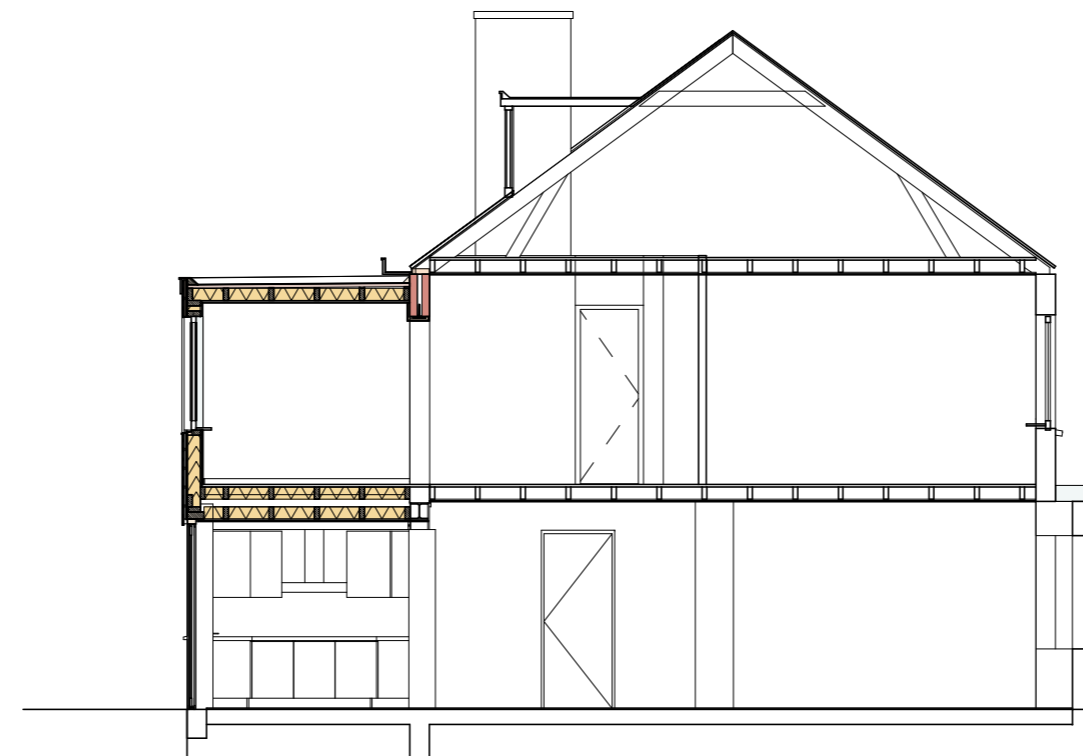
Doorsnede CC
