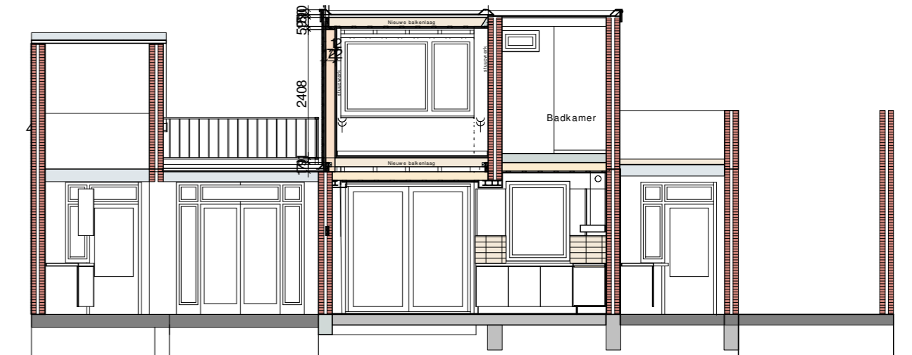
Doorsnede AA
