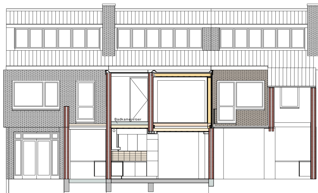
Doorsnede BB
